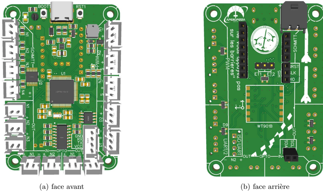
FIGURE 1.2 – Rendu 3D de la carte séquenceur
