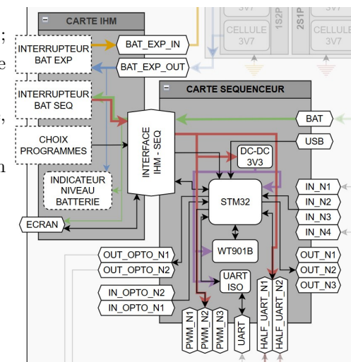
FIGURE 1.3 – Zoom sur le séquenceur et interface
